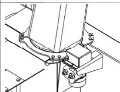
Rotation hydraulique, avec boyaux BER0078A
